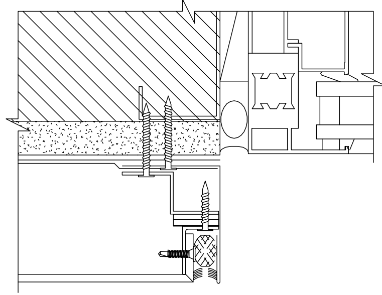
WINDOW / DOOR JAMB S10
